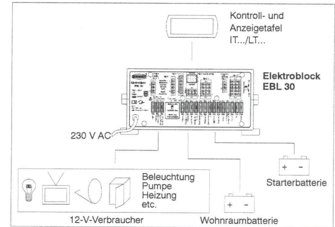
Bild 2 Energieversorgungssystem an Bord
