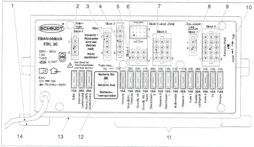
Bild 4 Aufbau Elektroblock EBL 30 (Front)
