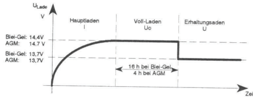
Bild 3 Ladespannungsverlauf mit dem Elektroblock EBL 30
