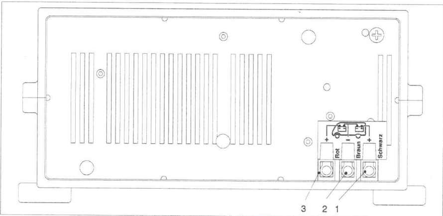
Bild 5 Aufbau Elektroblock EBL 30 (Rückseite)
