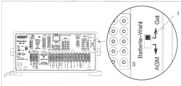
Bild 1 Batterie-Wahlschalter
